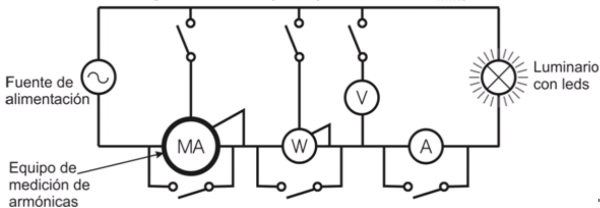
Figura A1. Circuito de prueba para luminarios con leds
